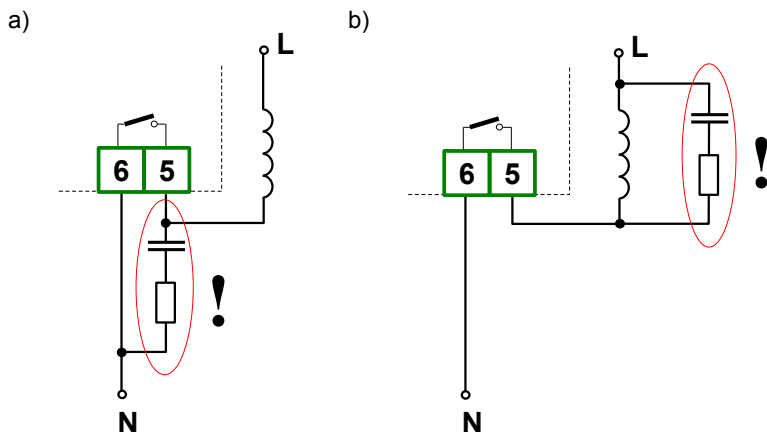
Rys. 4.16. Przykłady równoległego podłączenia obwodu tlumiącego: a) do styków przekaźnika; b) do obciążenia indukcyjnego
