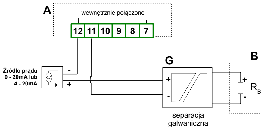
Rys. 4.22. Podłączenie przetwornika 2-przewodowego aktywnego z wyprowadzeniem sygnału prądowego do innego układu pomiarowego (np. sterownika PLC)
