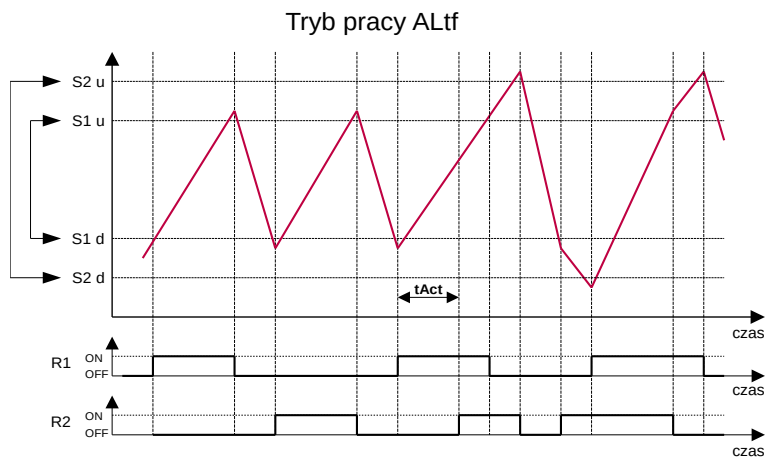
Rys. 6.7. Praca przekaźników w trybie ALtf – kontrola spadku wartości
