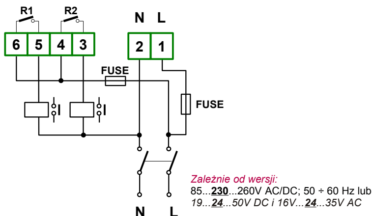
Rys. 4.15. Podłączenie zasilania oraz przekaźników sterujących obciążeniami
